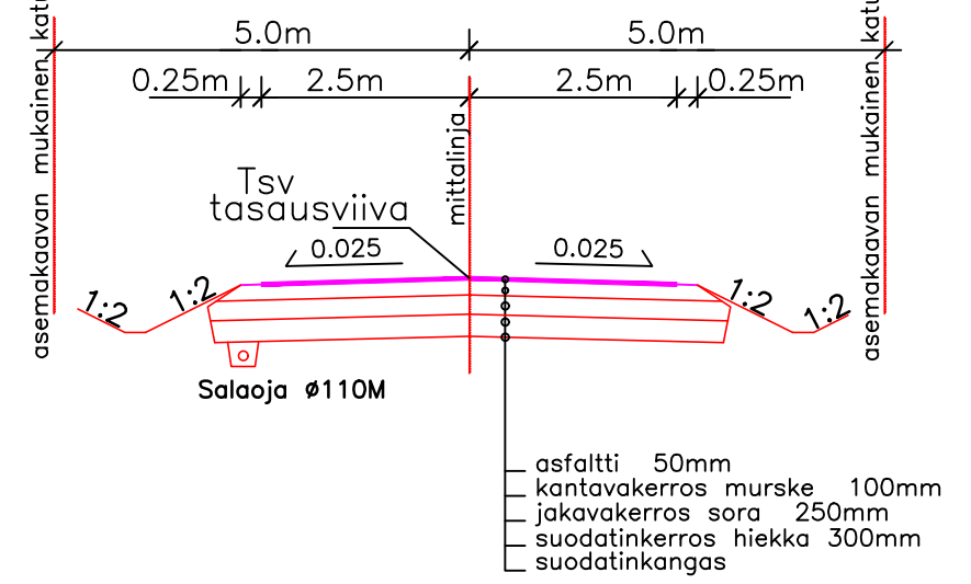
Tyypipoikkileikkaus:
