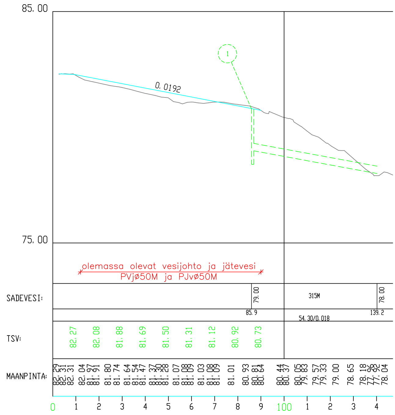
Pituusleikkaus:
